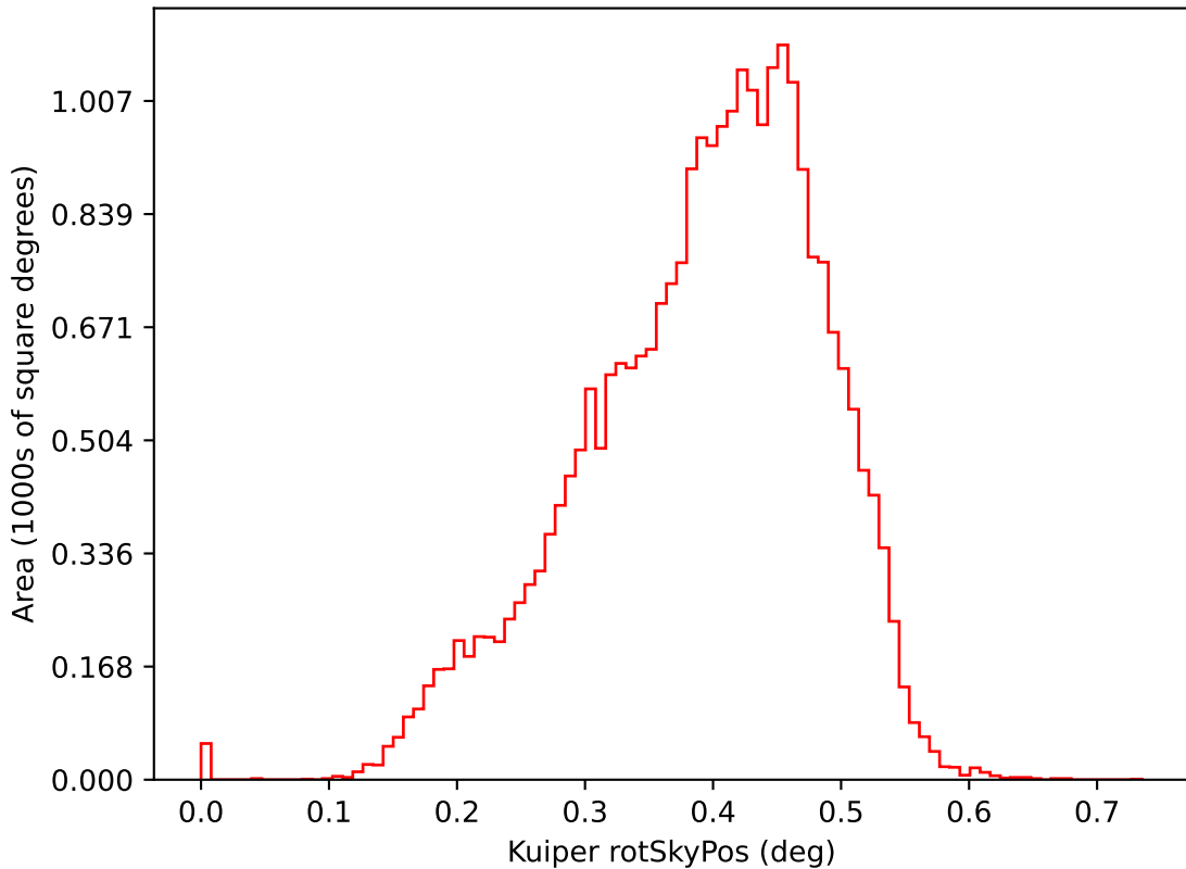
baseline_v2.0_10yrs i: Kuiper rotSkyPos
