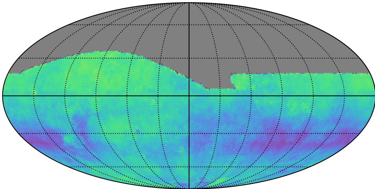
baseline_v2.0_10yrs i: Kuiper rotSkyPos
