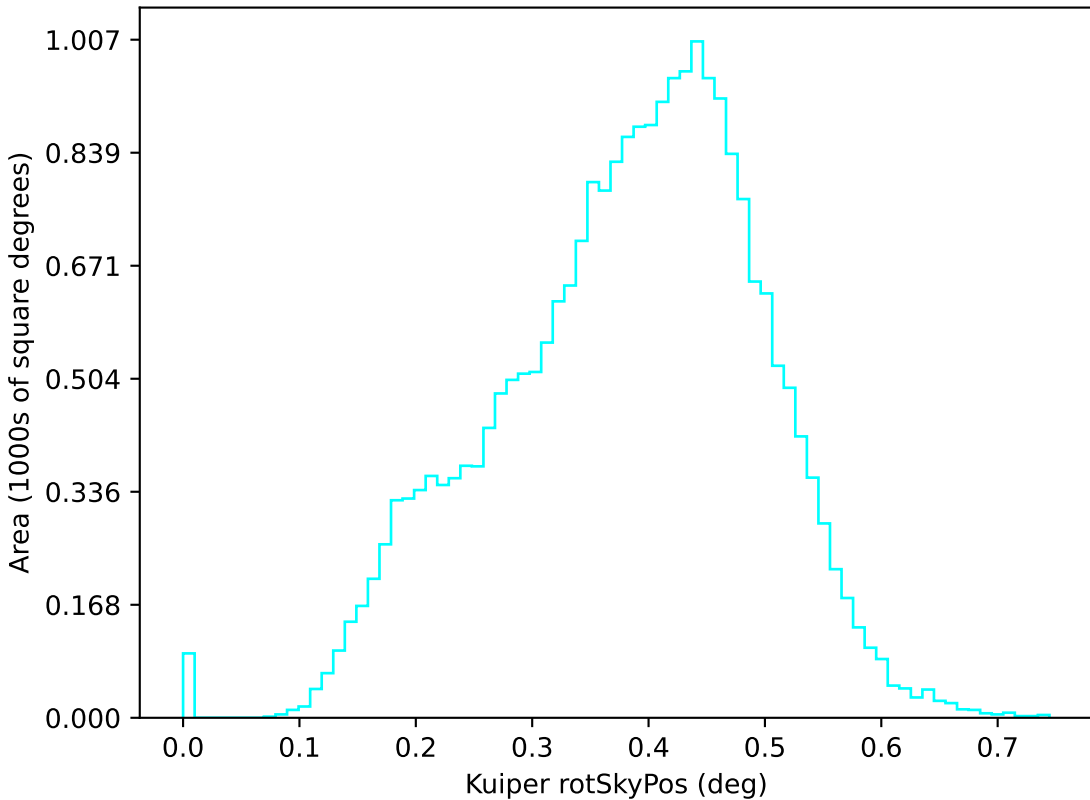
baseline_v2.0_10yrs u: Kuiper rotSkyPos
