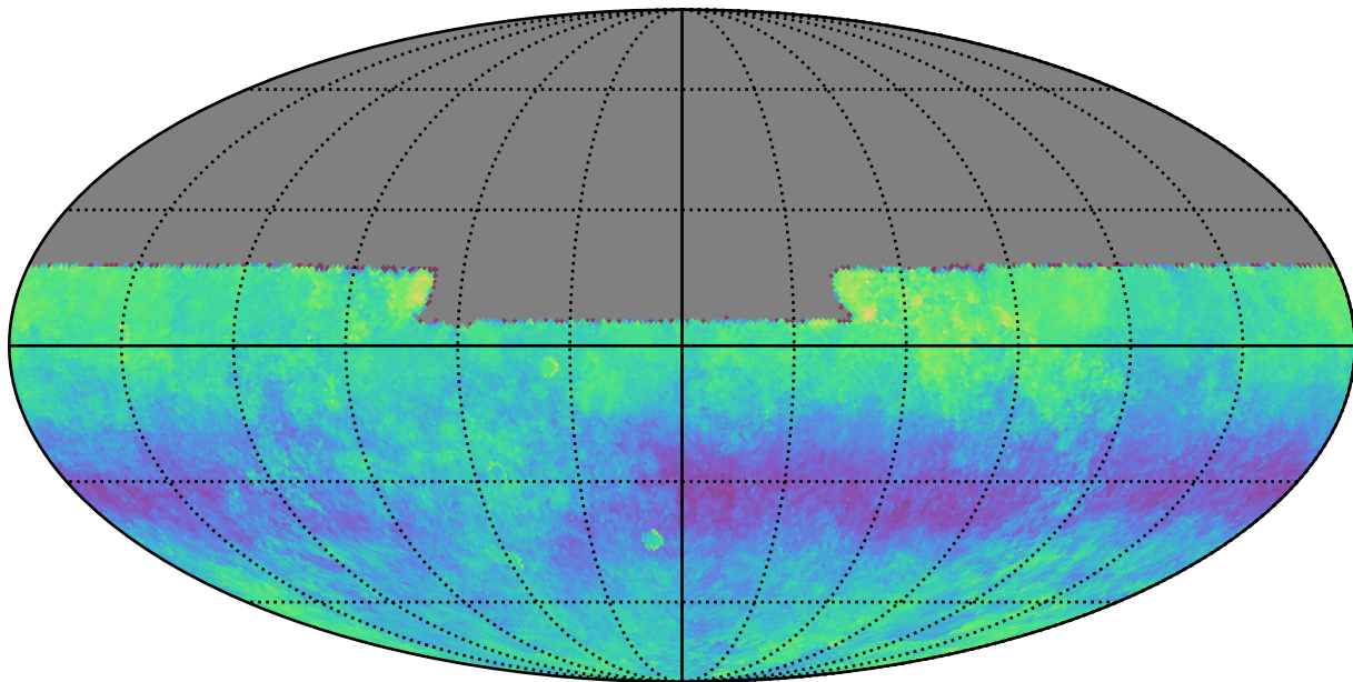
baseline_v2.0_10yrs u: Kuiper rotSkyPos
