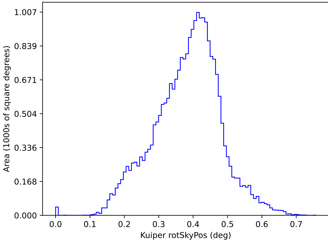
baseline_v2.0_10yrs y: Kuiper rotSkyPos
