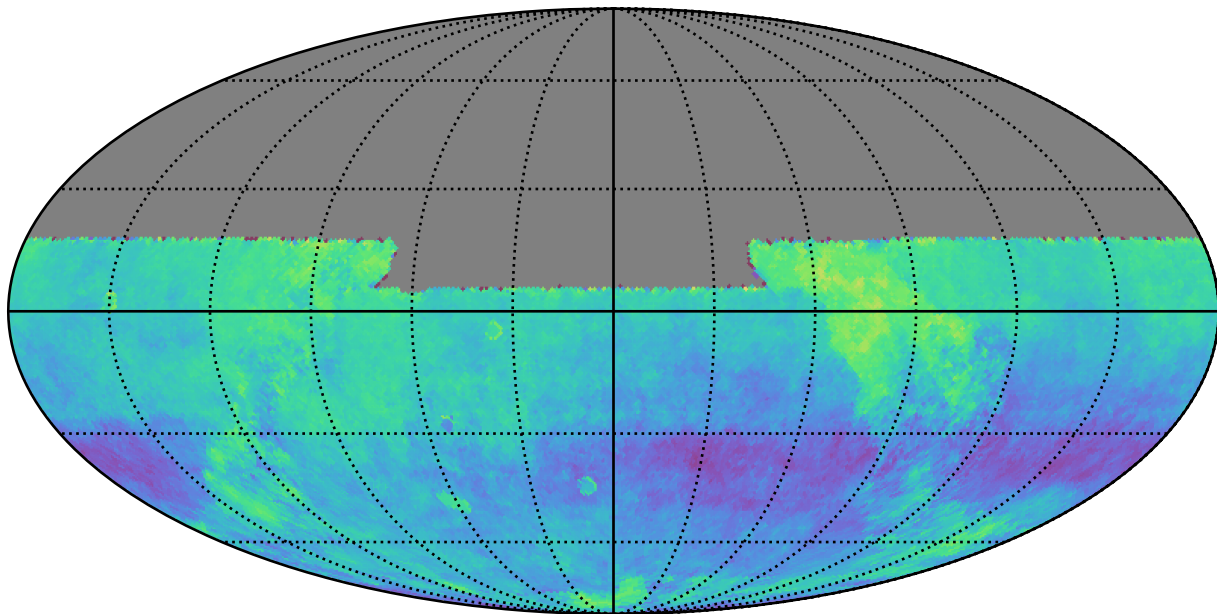
baseline_v2.0_10yrs y: Kuiper rotSkyPos
