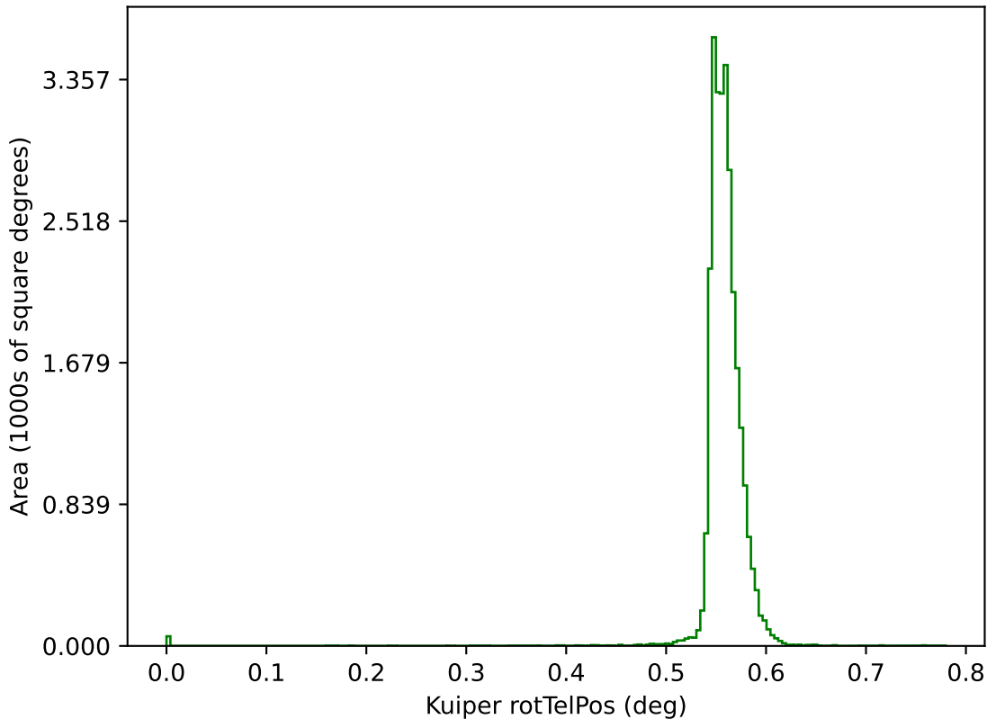
baseline_v2.0_10yrs g: Kuiper rotTelPos
