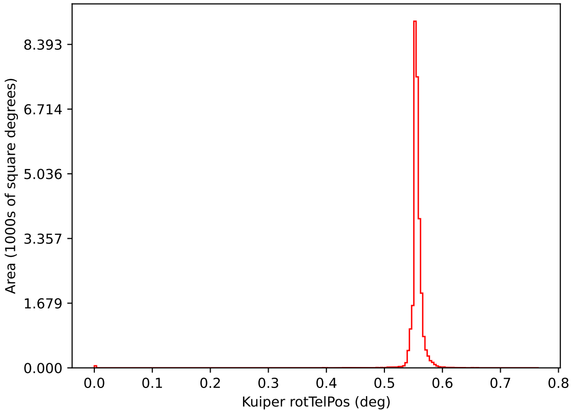
baseline_v2.0_10yrs i: Kuiper rotTelPos
