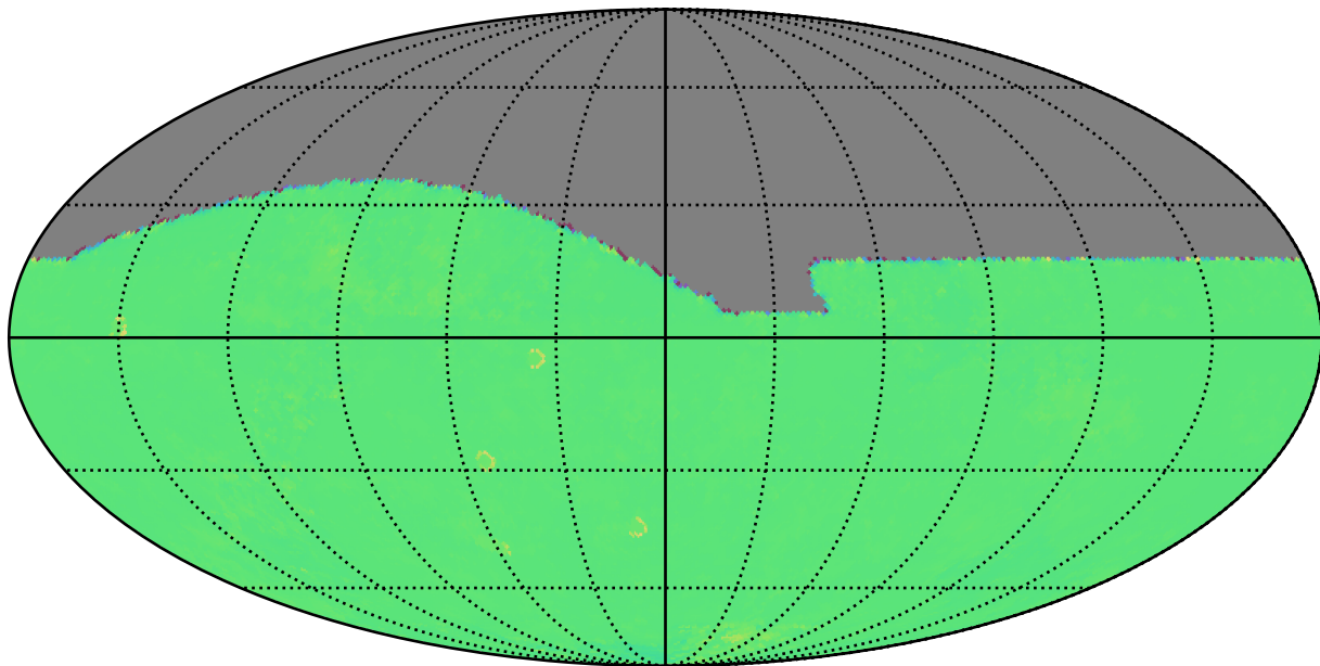
baseline_v2.0_10yrs i: Kuiper rotTelPos
