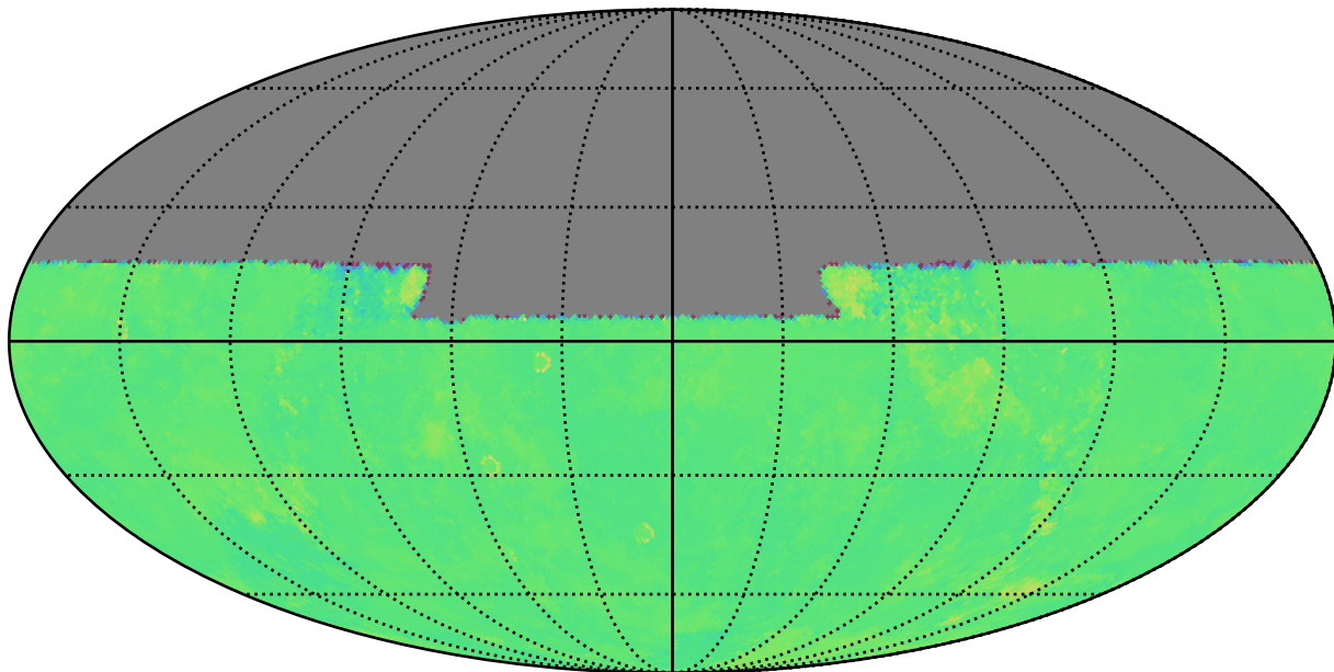
baseline_v2.0_10yrs u: Kuiper rotTelPos
