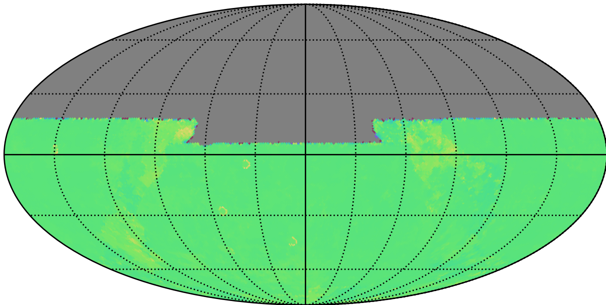
baseline_v2.0_10yrs y: Kuiper rotTelPos
