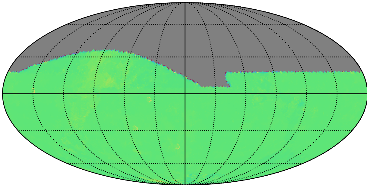
baseline_v2.0_10yrs z: Kuiper rotTelPos
