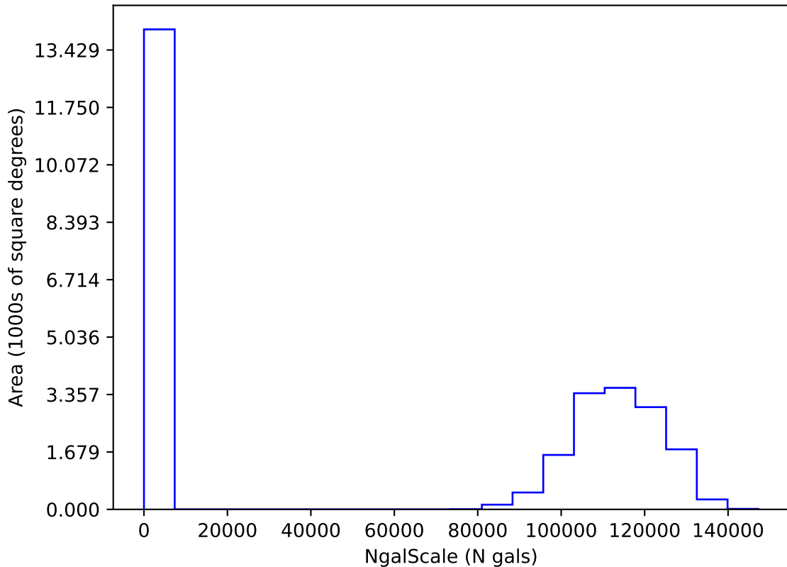
baseline_v2.0_10yrs i: NgalScale
