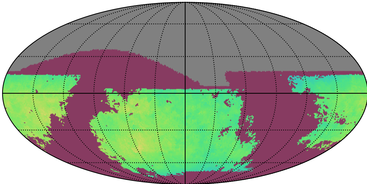
baseline_v2.0_10yrs i: NgalScale
