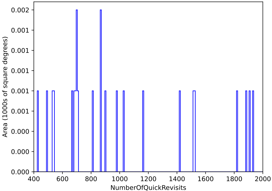
baseline_v2.0_10yrs : NumberOfQuickRevisits
