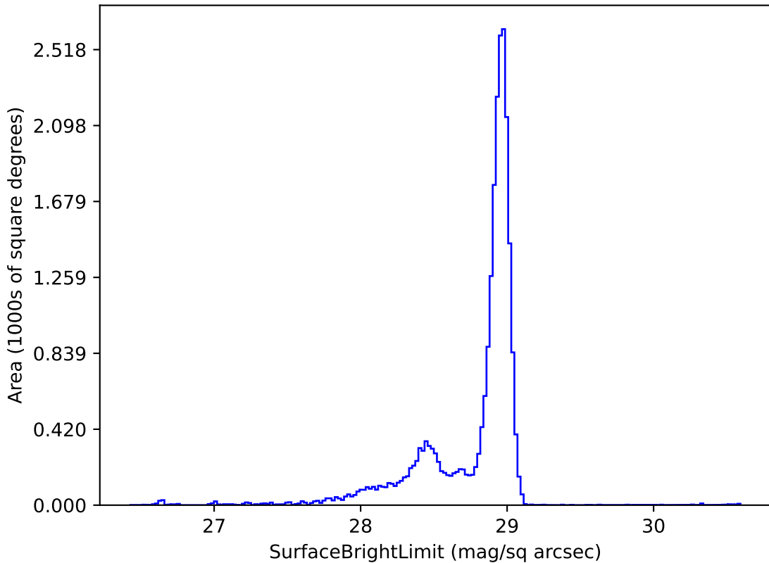
baseline_v2.0_10yrs u: SurfaceBrightLimit
