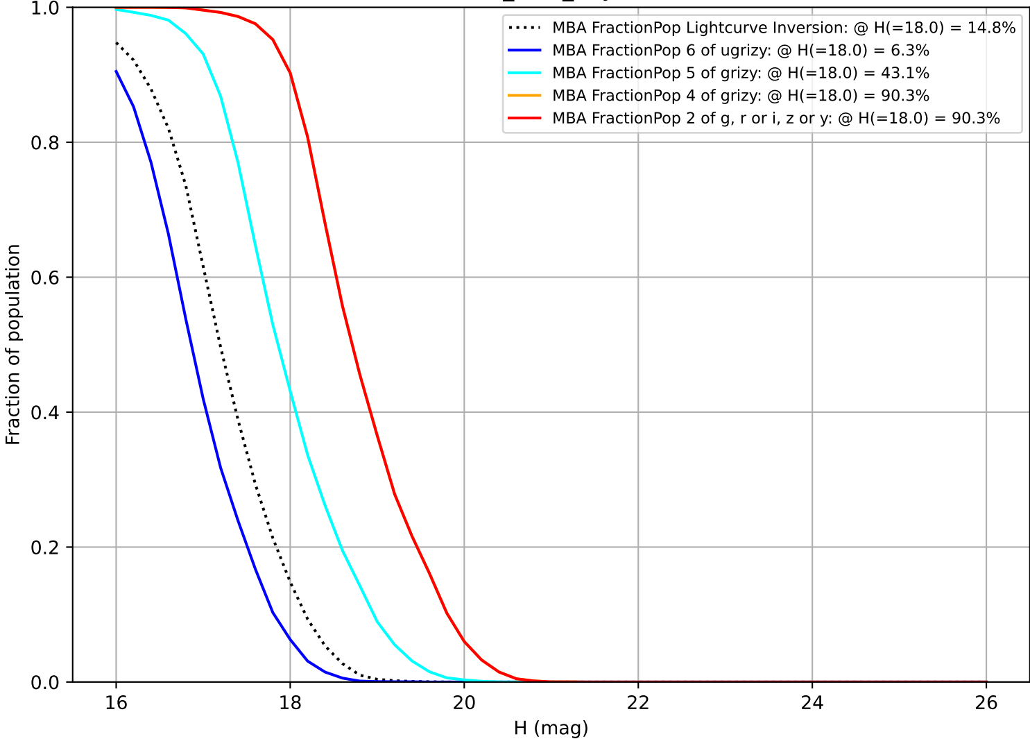
baseline_v2.0_10yrs MBA
