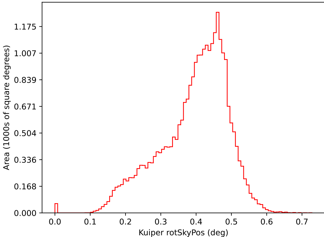
baseline_v2.1_10yrs i: Kuiper rotSkyPos
