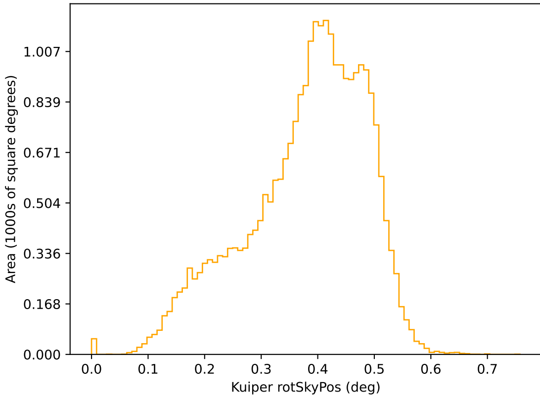
baseline_v2.1_10yrs r: Kuiper rotSkyPos
