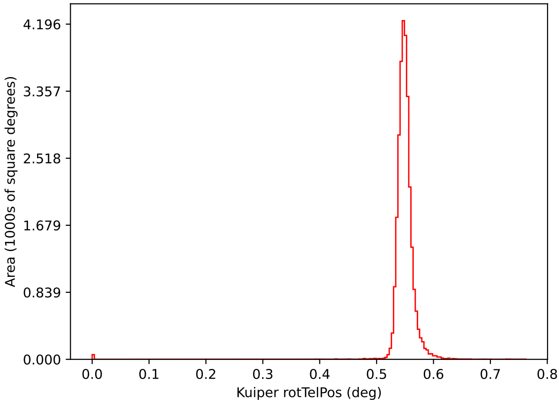
baseline_v2.1_10yrs i: Kuiper rotTelPos
