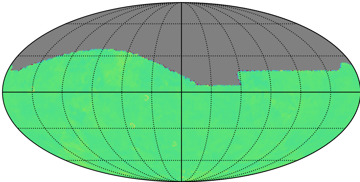
baseline_v2.1_10yrs r: Kuiper rotTelPos
