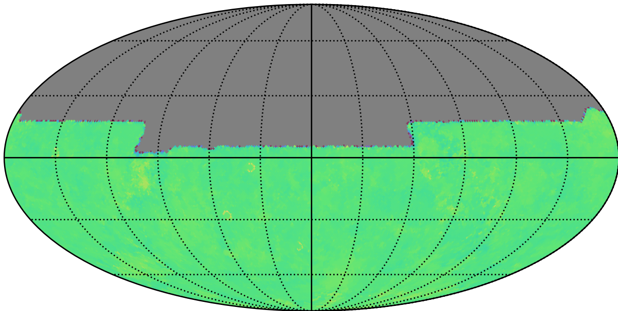
baseline_v2.1_10yrs u: Kuiper rotTelPos
