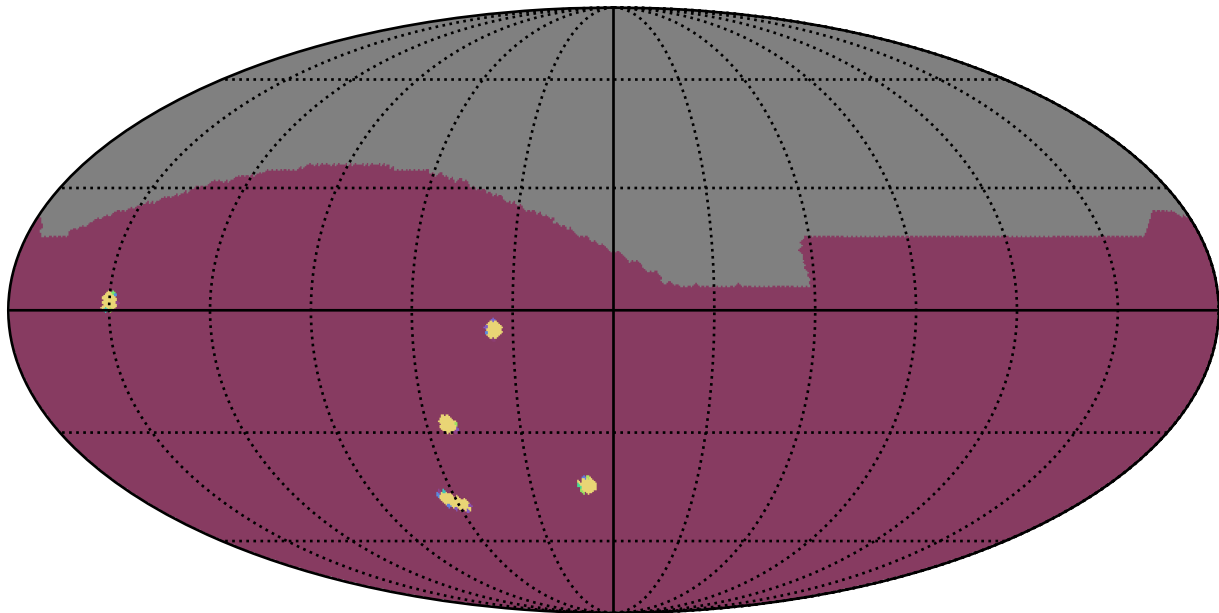
baseline_v2.1_10yrs : NumberOfQuickRevisits
