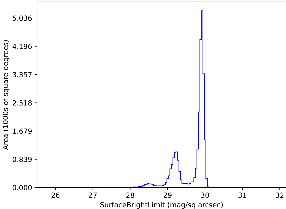
baseline_v2.1_10yrs i: SurfaceBrightLimit
