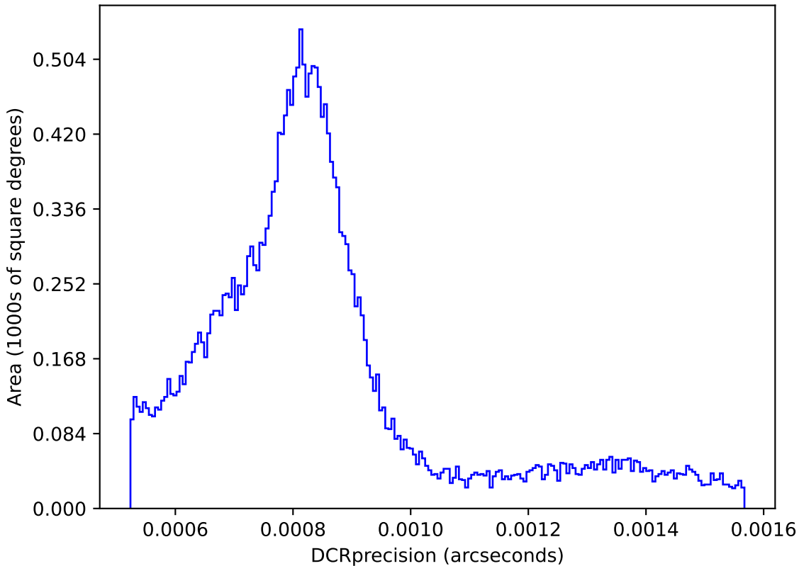
baseline_v2.2_10yrs : DCRprecision
