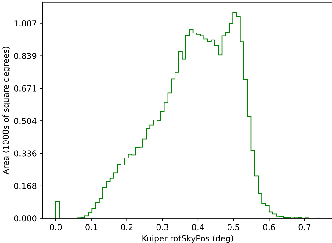
baseline_v2.2_10yrs g: Kuiper rotSkyPos
