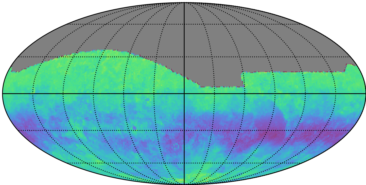
baseline_v2.2_10yrs g: Kuiper rotSkyPos
