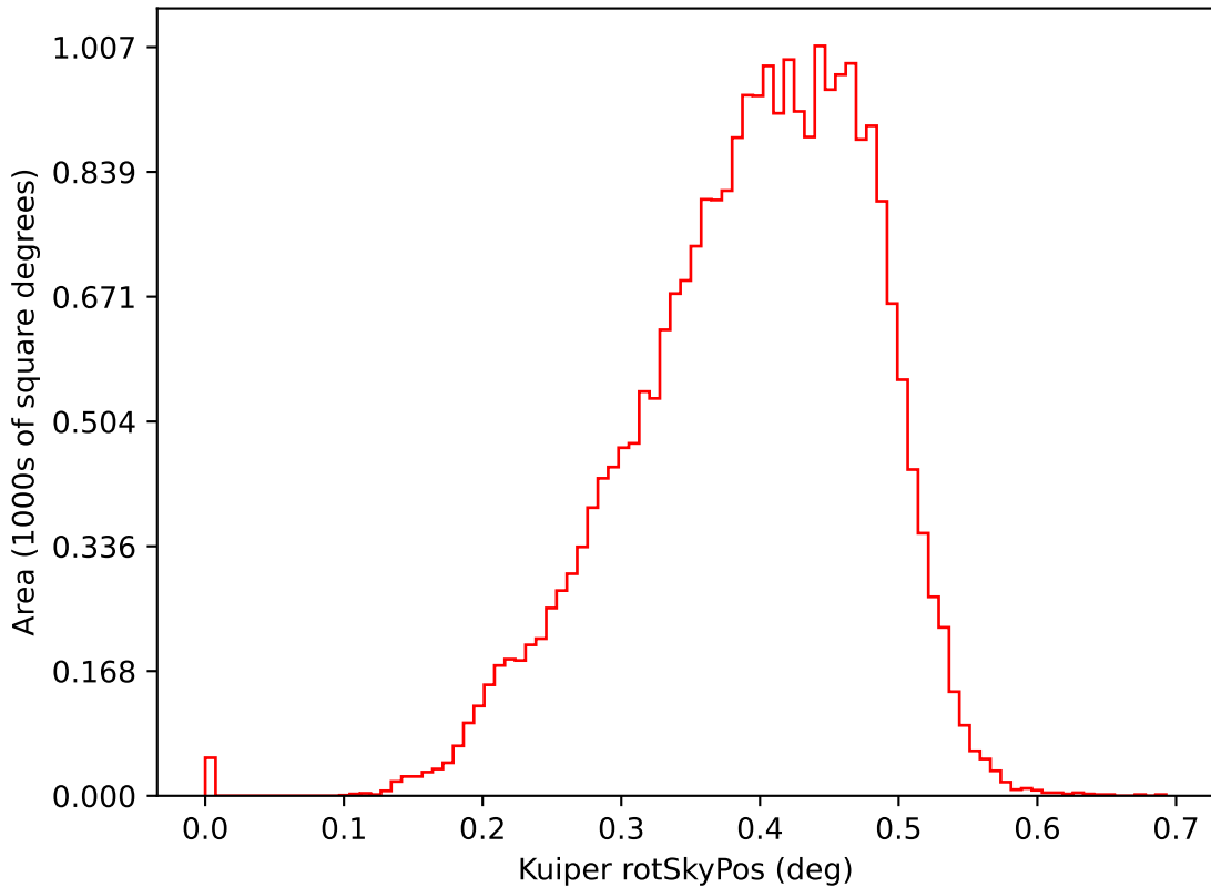
baseline_v2.2_10yrs i: Kuiper rotSkyPos
