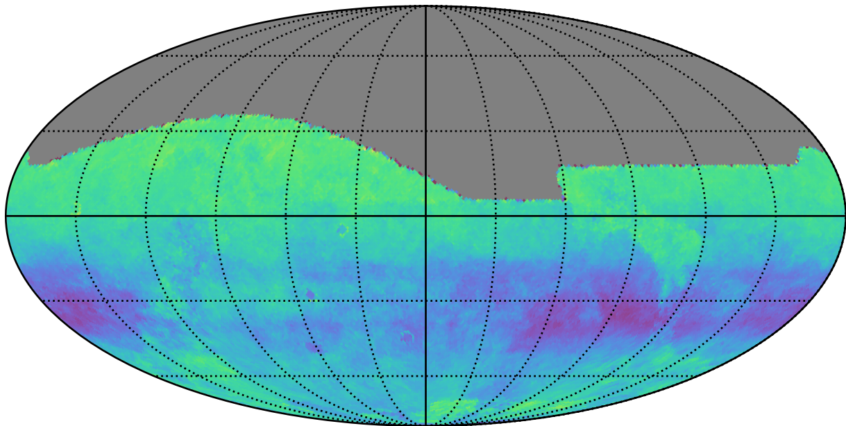
baseline_v2.2_10yrs r: Kuiper rotSkyPos
