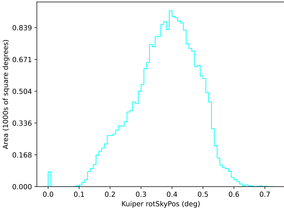
baseline_v2.2_10yrs u: Kuiper rotSkyPos
