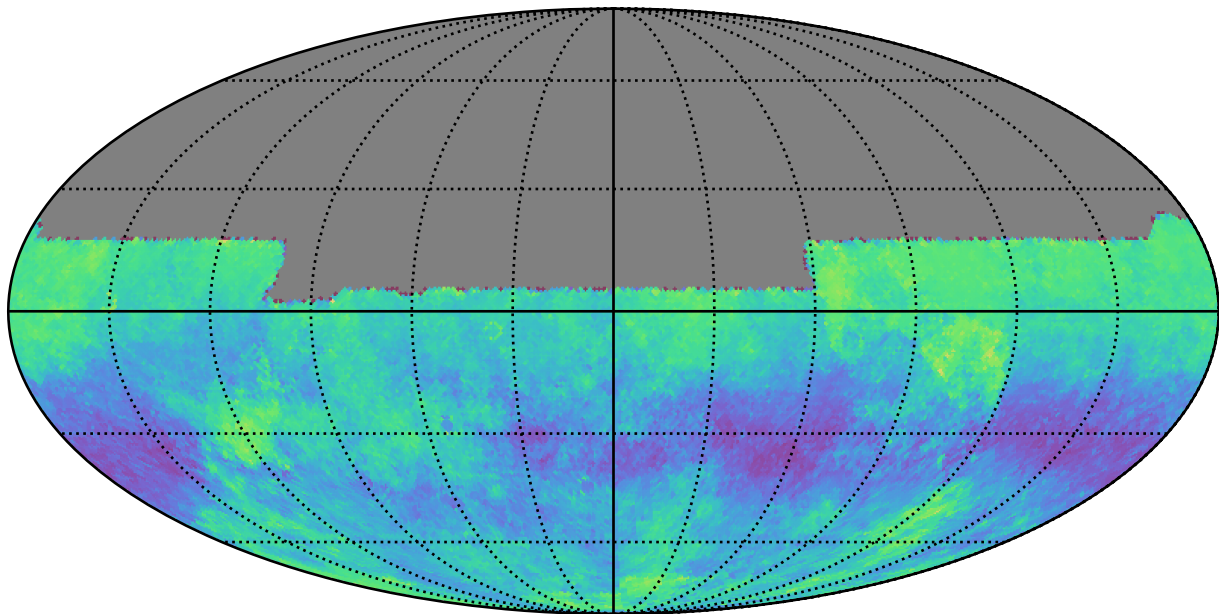
baseline_v2.2_10yrs u: Kuiper rotSkyPos
