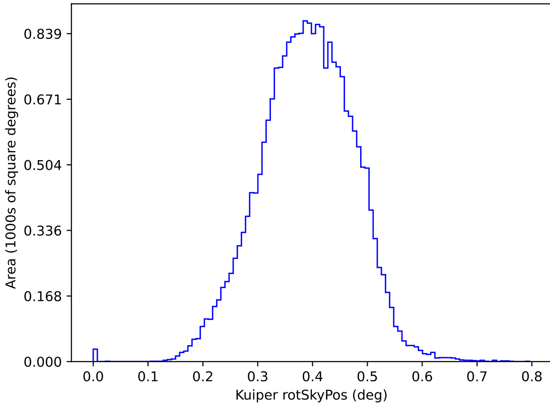
baseline_v2.2_10yrs y: Kuiper rotSkyPos
