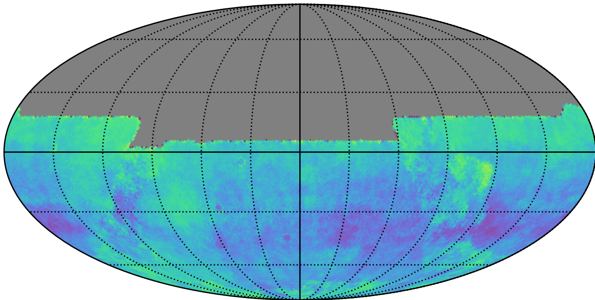
baseline_v2.2_10yrs y: Kuiper rotSkyPos
