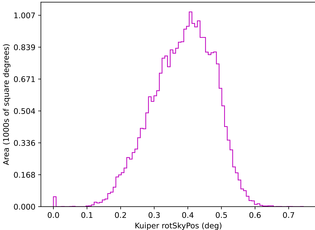
baseline_v2.2_10yrs z: Kuiper rotSkyPos
