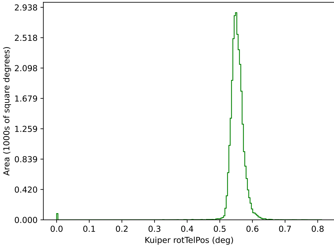
baseline_v2.2_10yrs g: Kuiper rotTelPos
