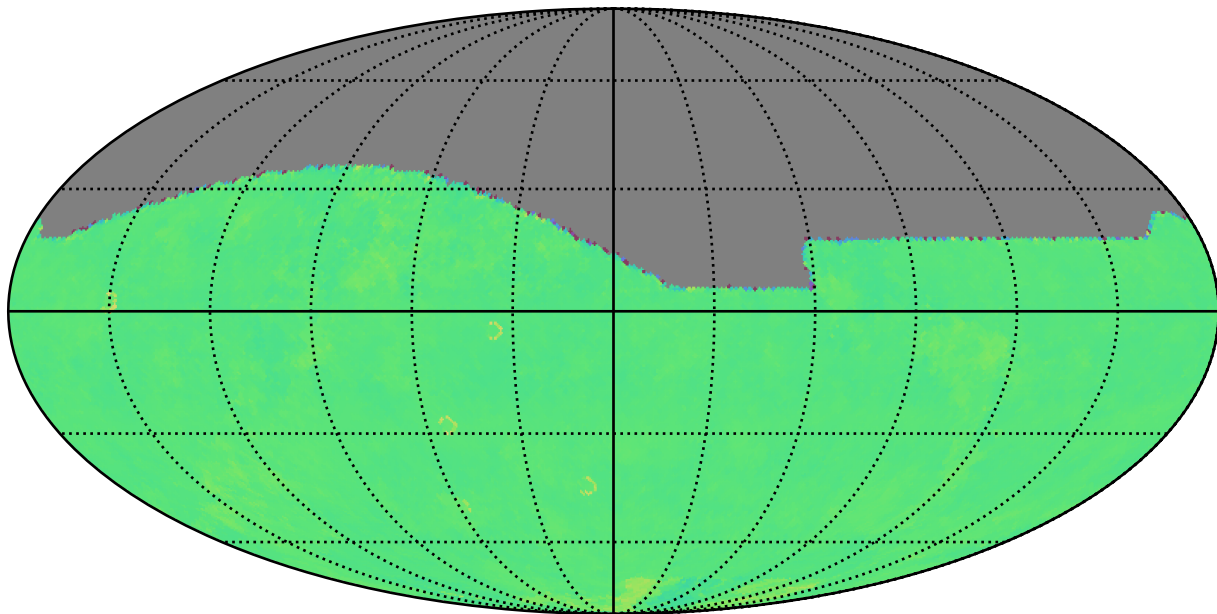
baseline_v2.2_10yrs r: Kuiper rotTelPos
