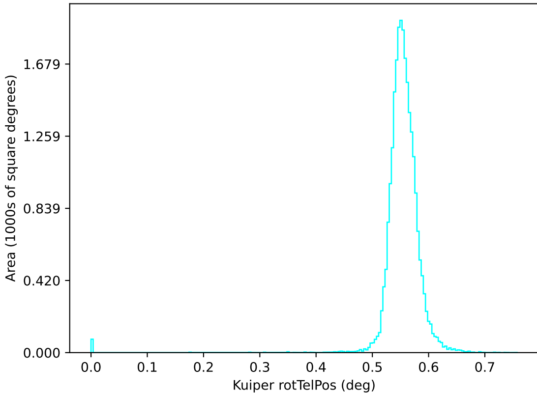
baseline_v2.2_10yrs u: Kuiper rotTelPos
