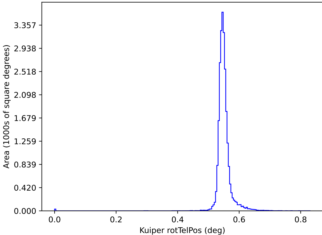
baseline_v2.2_10yrs y: Kuiper rotTelPos
