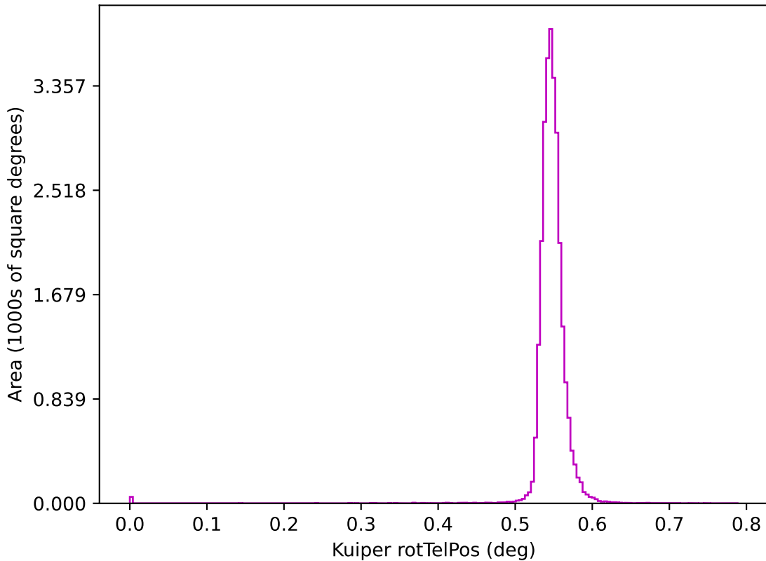
baseline_v2.2_10yrs z: Kuiper rotTelPos
