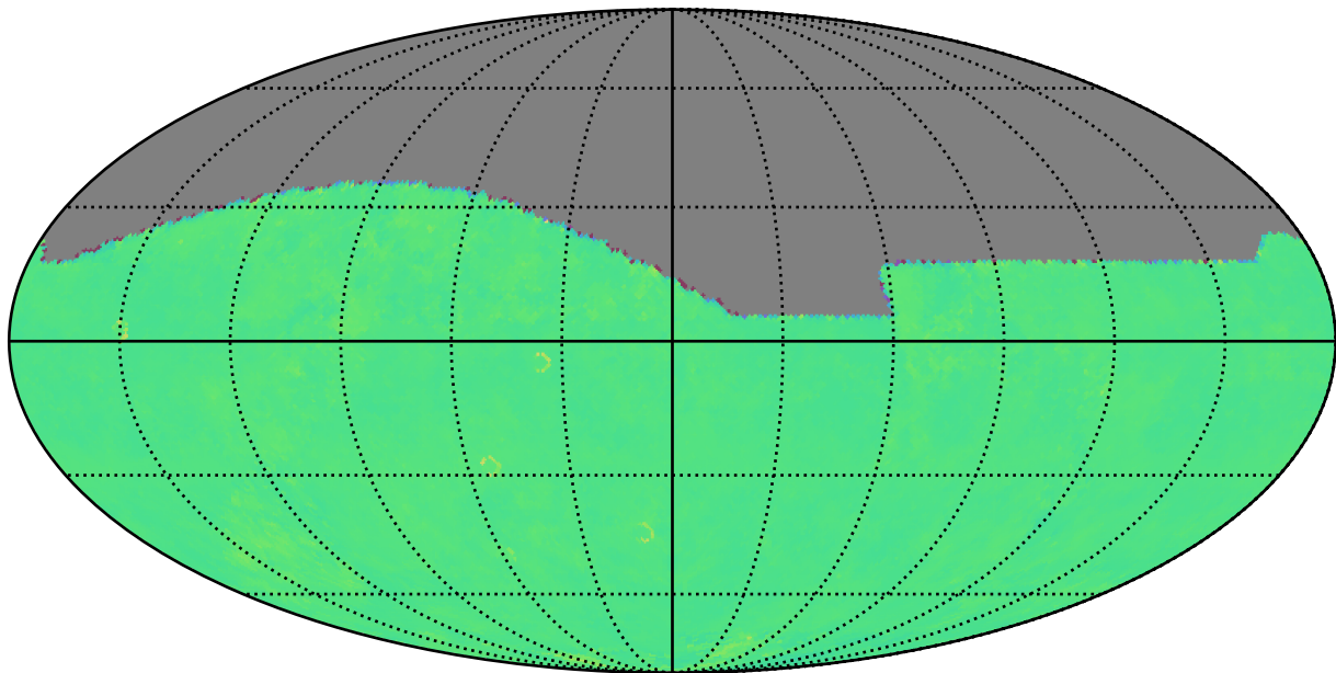
baseline_v2.2_10yrs z: Kuiper rotTelPos
