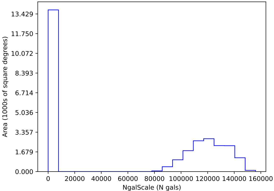
baseline_v2.2_10yrs i: NgalScale
