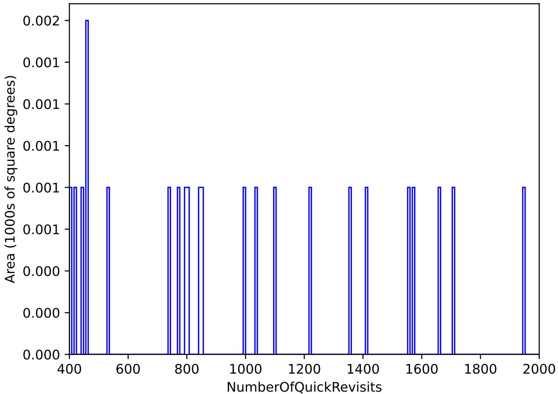
baseline_v2.2_10yrs : NumberOfQuickRevisits
