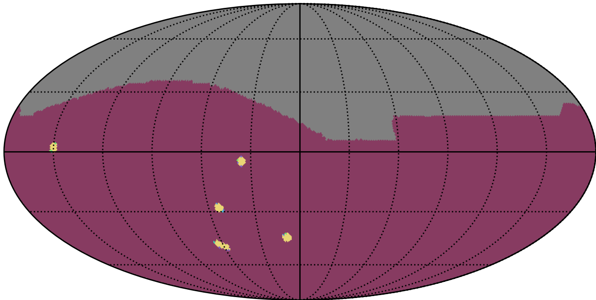
baseline_v2.2_10yrs : NumberOfQuickRevisits
