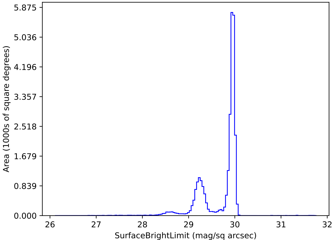
baseline_v2.2_10yrs i: SurfaceBrightLimit
