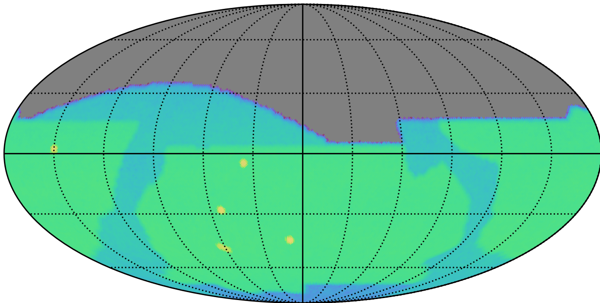
baseline_v2.2_10yrs i: SurfaceBrightLimit
