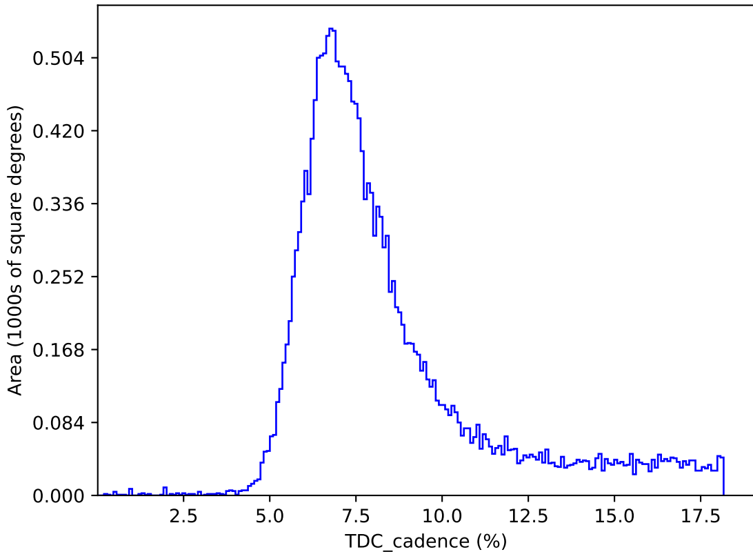
baseline_v2.2_10yrs : TDC_cadence
