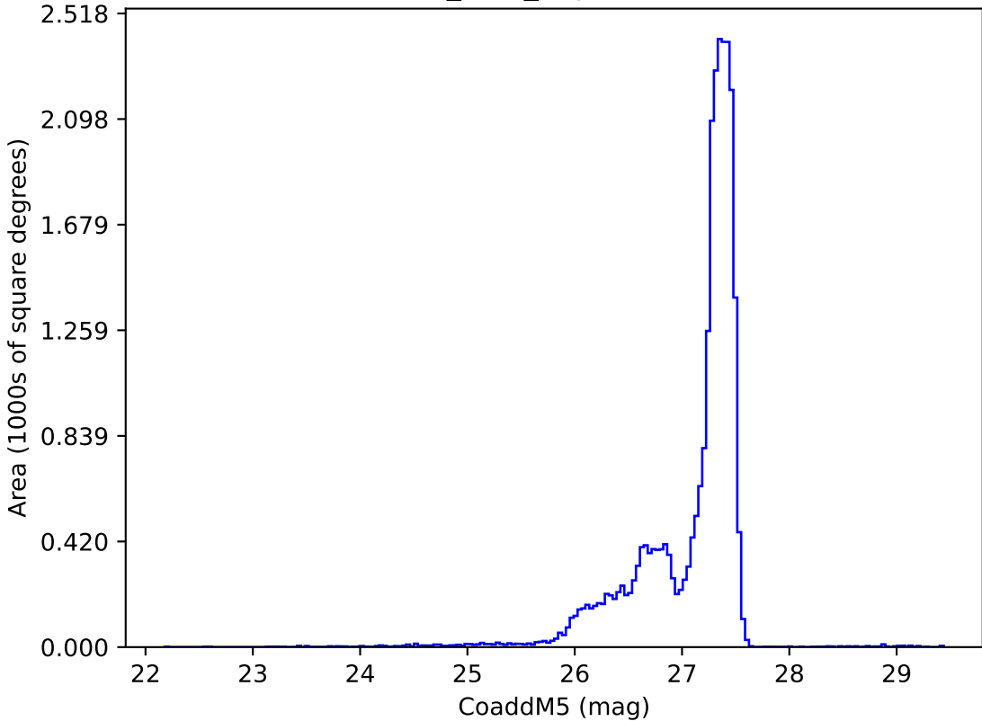
baseline_v3.0_10yrs : CoaddM5
