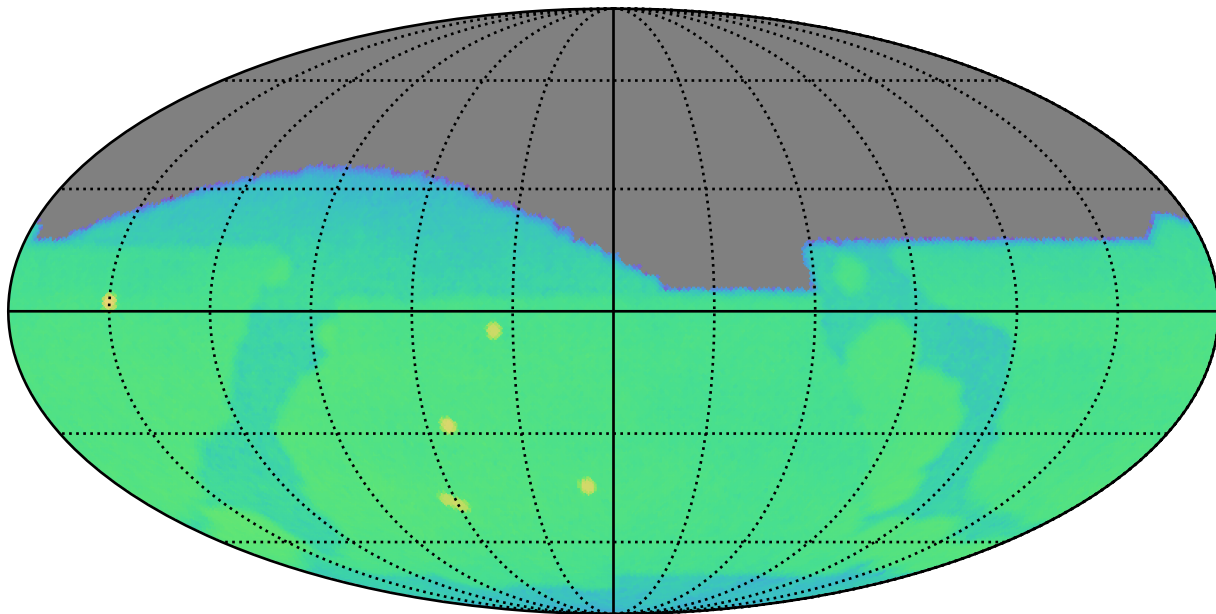
baseline_v3.0_10yrs g: CoaddM5
