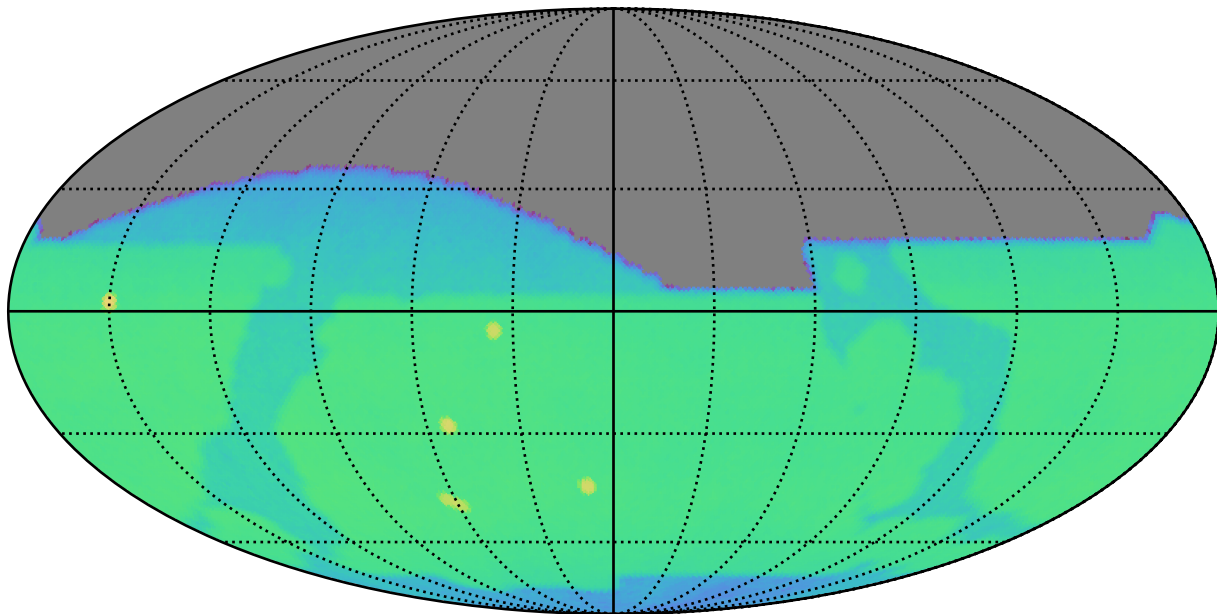
baseline_v3.0_10yrs i: CoaddM5
