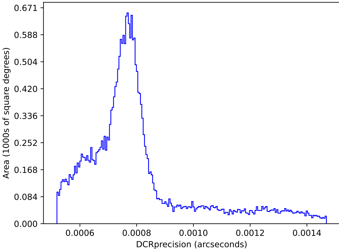
baseline_v3.0_10yrs : DCRprecision
